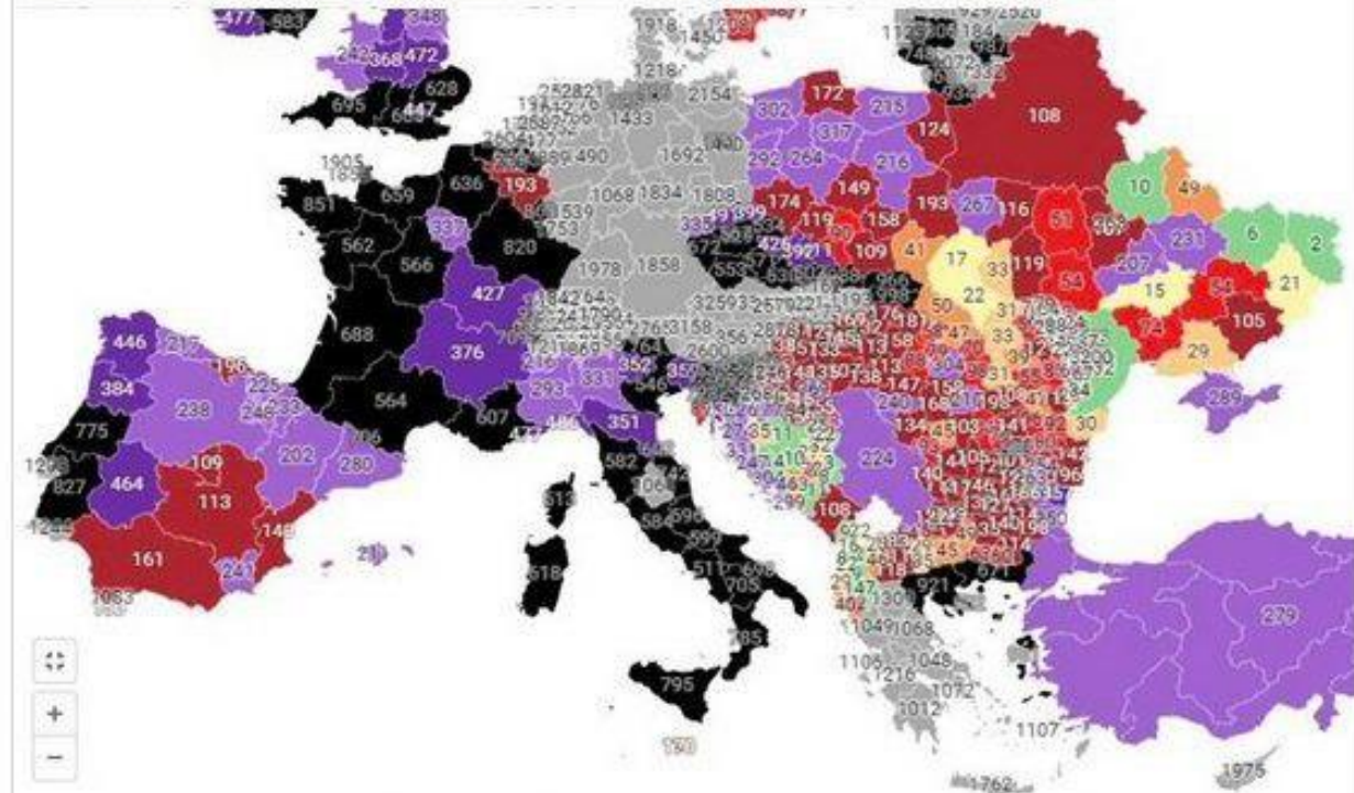
Europa Corona 7-Tage-Inzidenz pro Region - 11. März 2022
