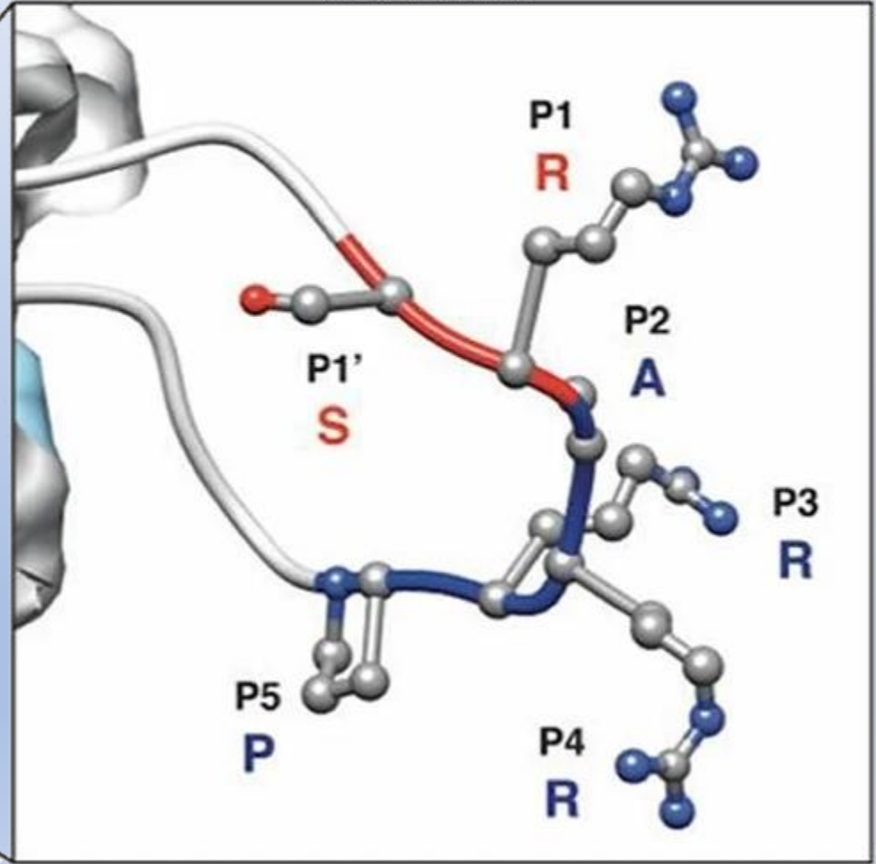
S1/S2 site
