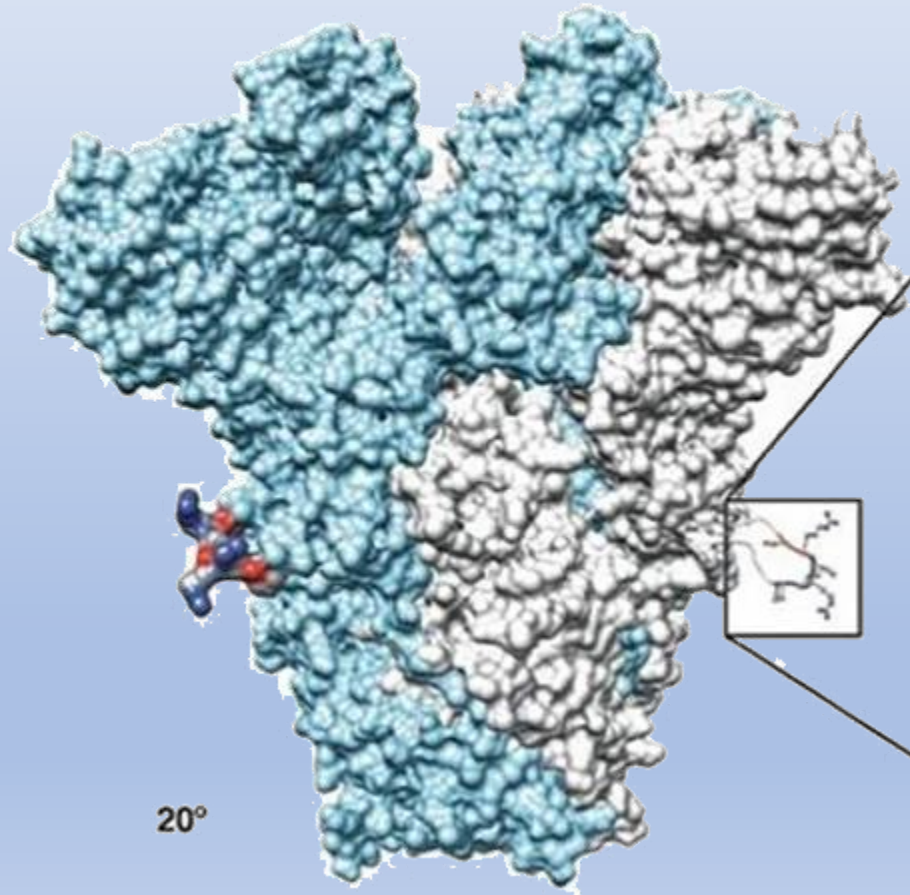
SARS-CoV-2
