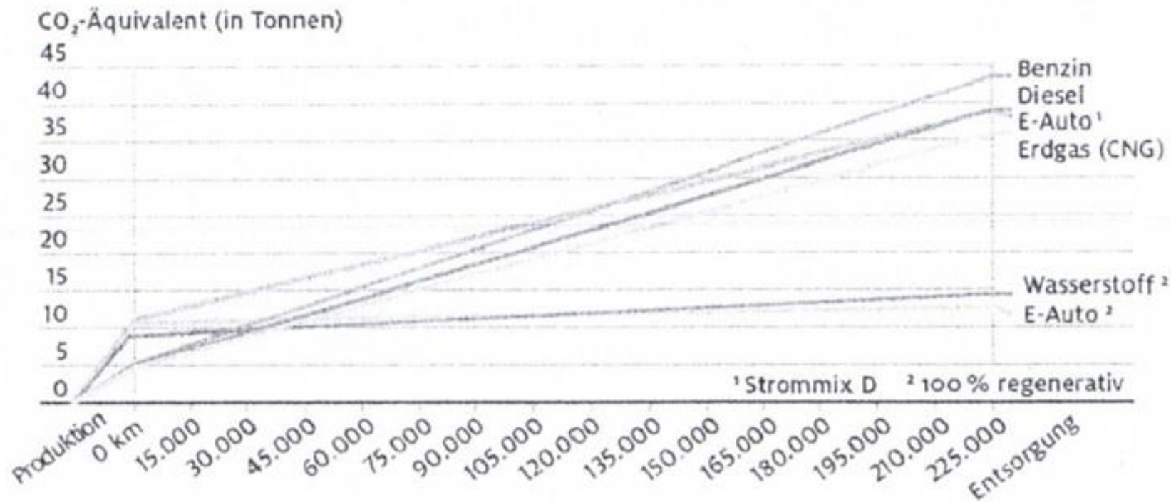
Figuur 1 Vergelijking CO 2 -uitstoot op basis van type aandrijving (ADAC, 2019)
